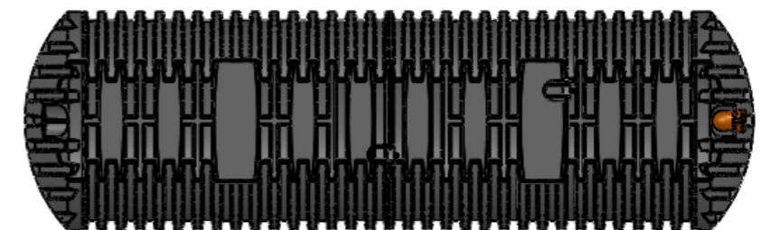
SECTION D-D SCALE 1 : 55
